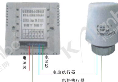
水地暖（常闭型）接线方式
