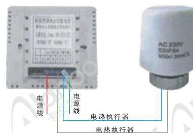
水地暖（常开型）接线方式
